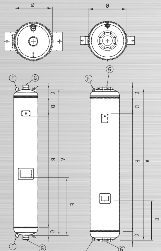
FLANGIATO-FLANGED
